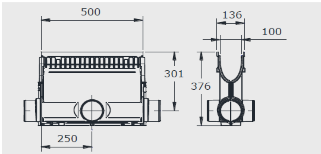
1 pav. Itekėjimo dėžės gabaritiniai matmenys
