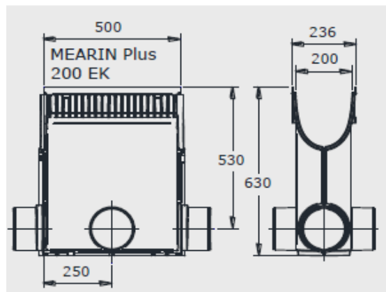
1 pav. Iškėjimo dėžės gabaritiniai matmenys
